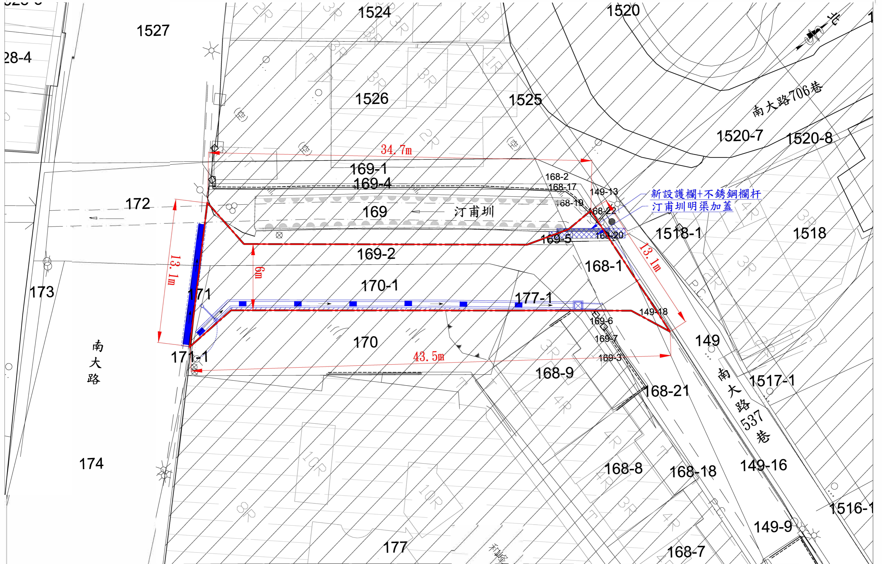
新竹市南大路537巷口6公尺道路拓寬工程平面配置圖3-3
