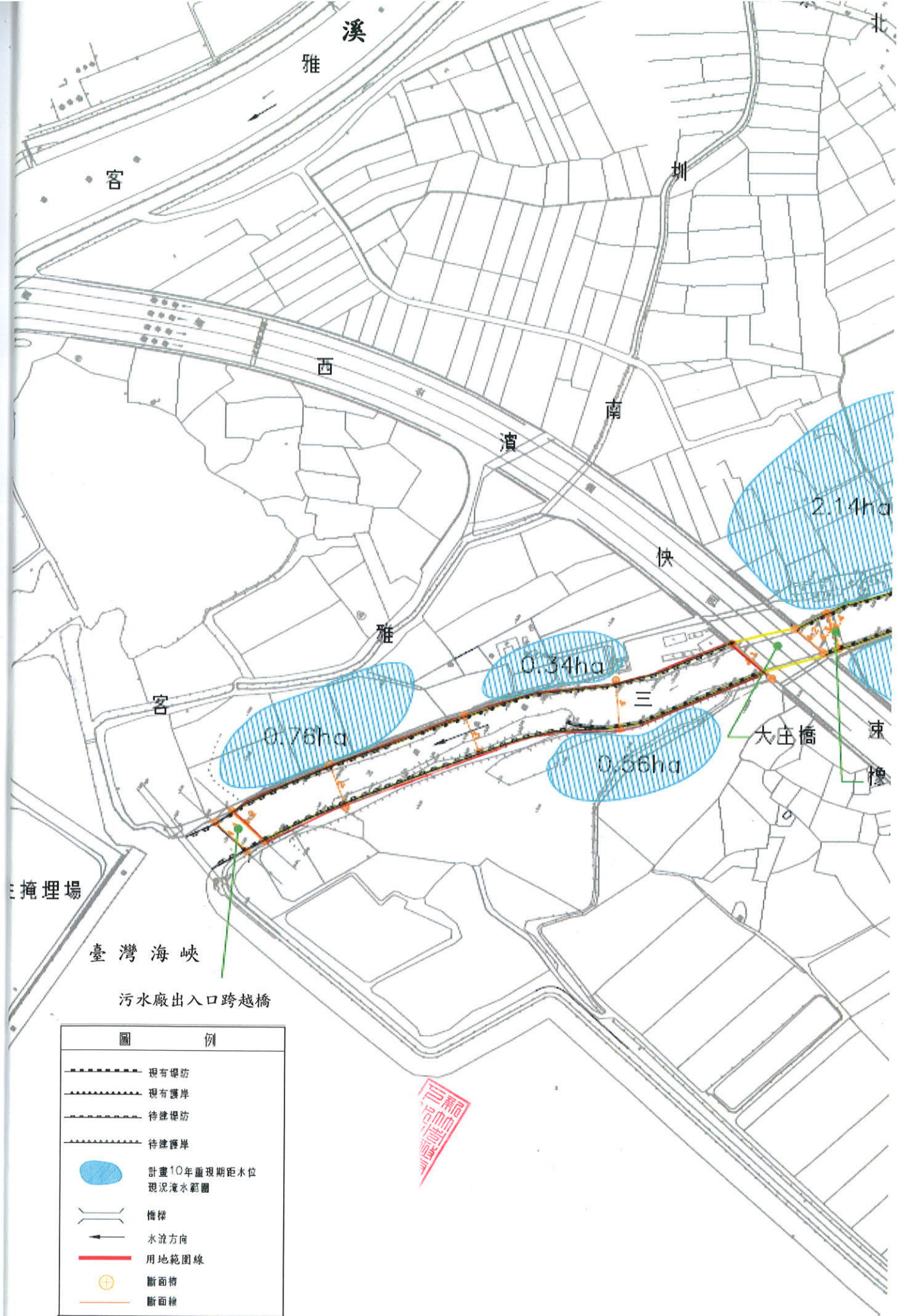
三姓溪出海口段堤防工程(0K+000~0K+500)土地使用計畫圖
