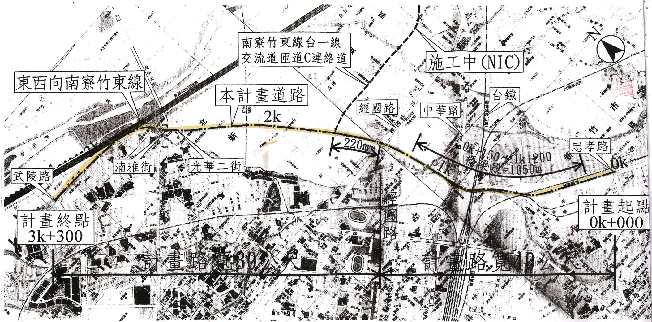
新竹市公道五延伸新闢道路(向西)工程徵收土地使用計畫圖
